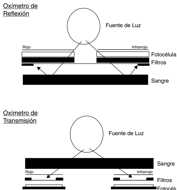
Figura 2 Principio de la oximetría de transmisión y reflexión. Fuente: Mellerowicz 4 .
